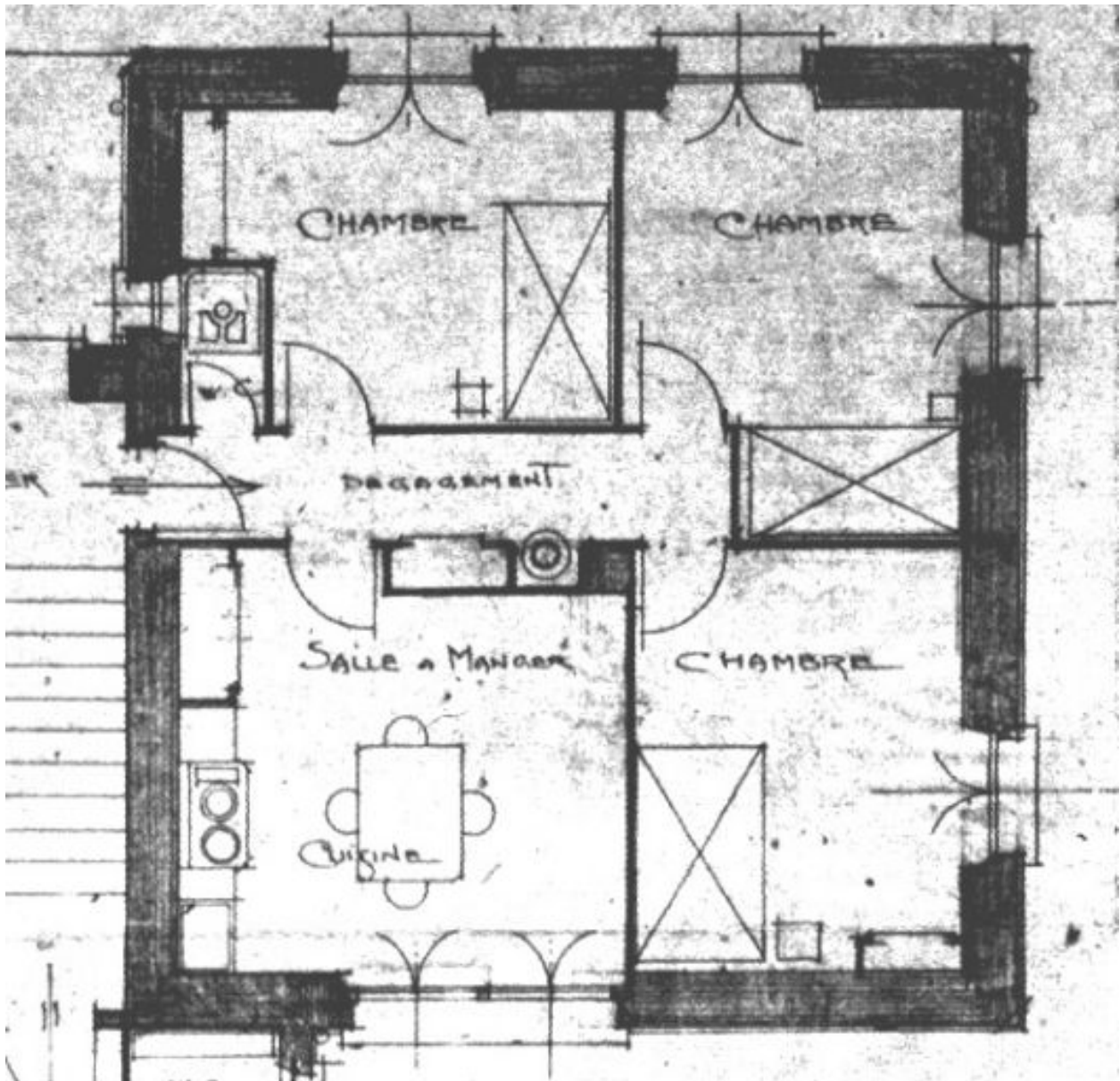
Plan d'un appartement de 4 pièces. Extrait du plan d'ensemble / 30 mars 1912 (AC Lyon : 0002 S 01119)
