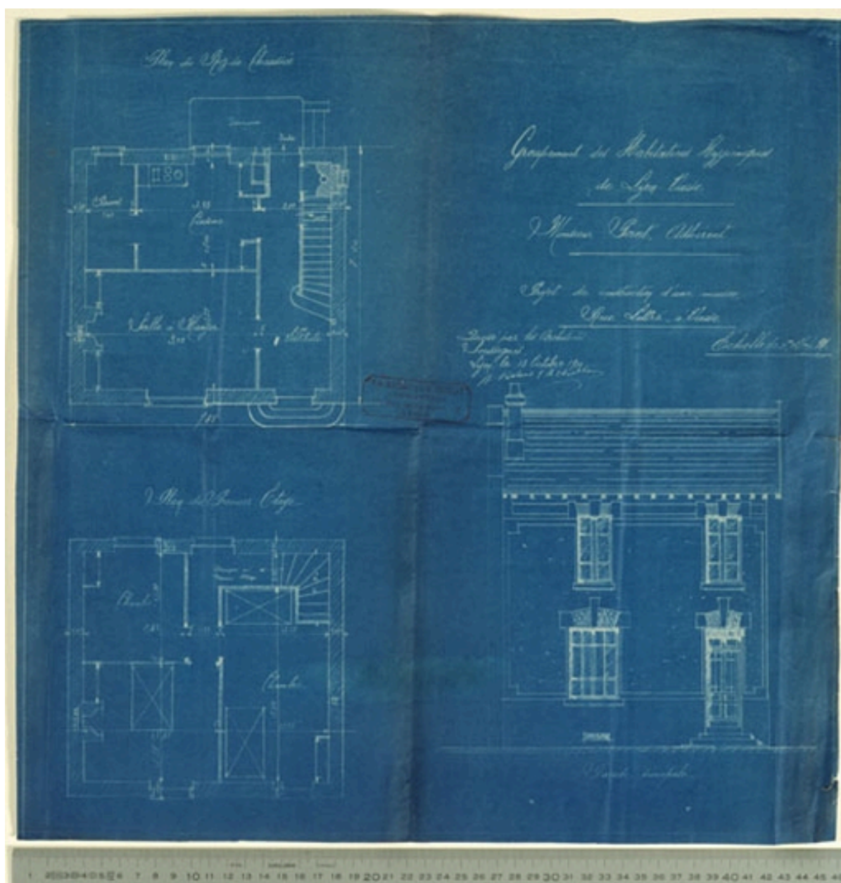
314 WP 1910 permis 906, plans, façade d'une maison individuelle au 12 rue Littré
