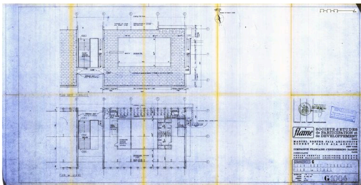
Commerces G. Plans du 1er étage et du toit-terrasse. Marcel Breuer, Robert F. Gatje, 13 décembre 1962 (AC Arâches-la-Frasse)
