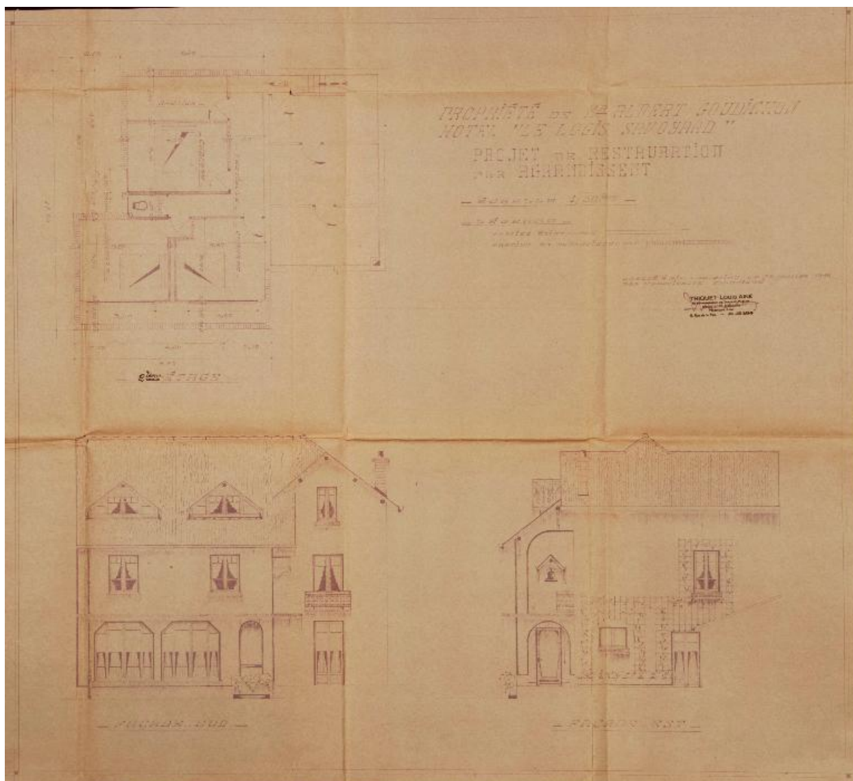
Plan du 2e étage, façades est et sud, 1946
