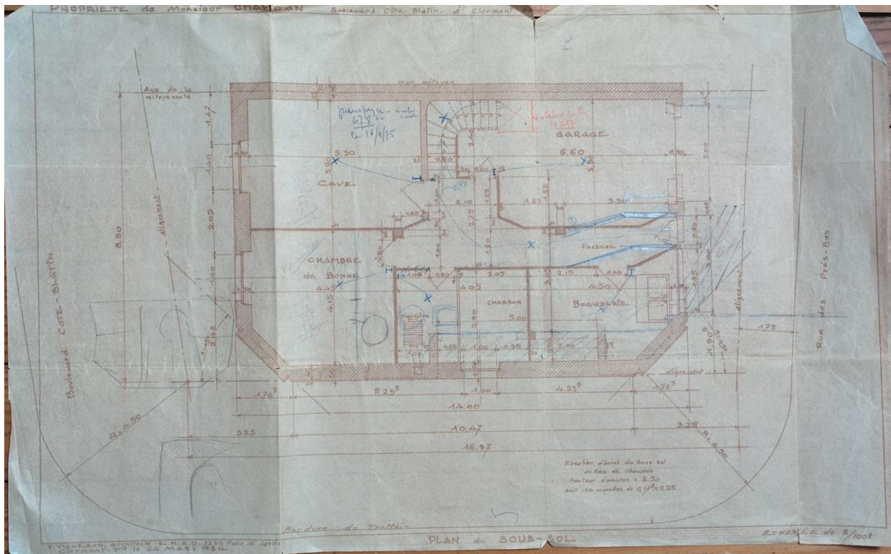
Plan du sous-sol (plans modificatifs 1934)
