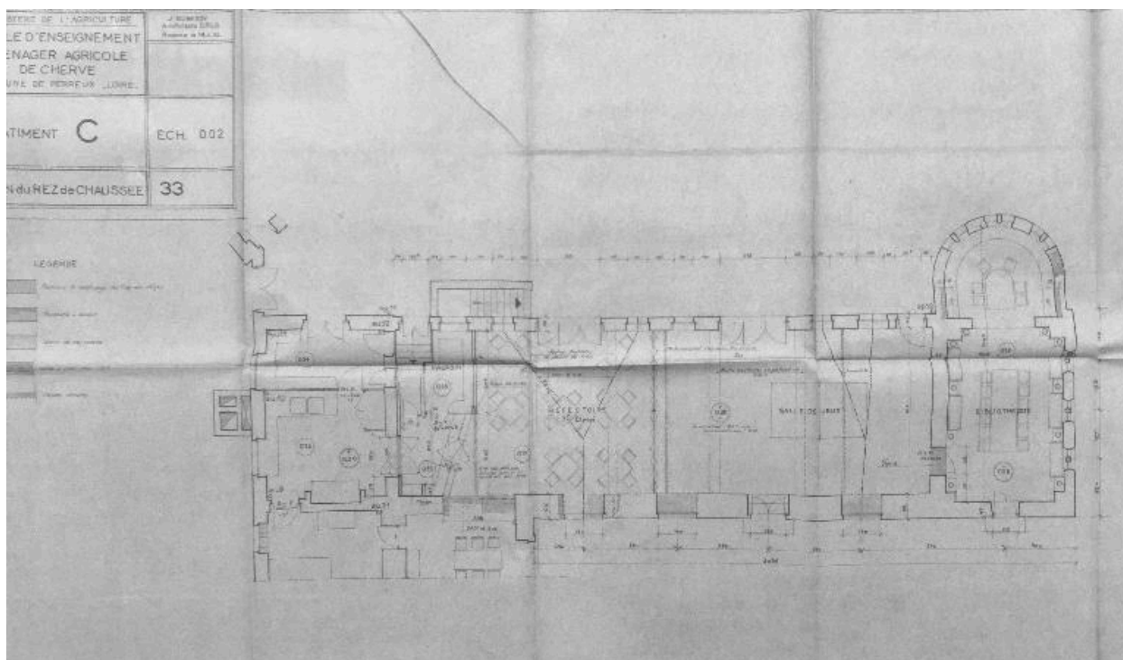
Château, corps de bâtiment C : plan du rez-de-chaussée, 1955 (AD Loire, 690 VT 39)
