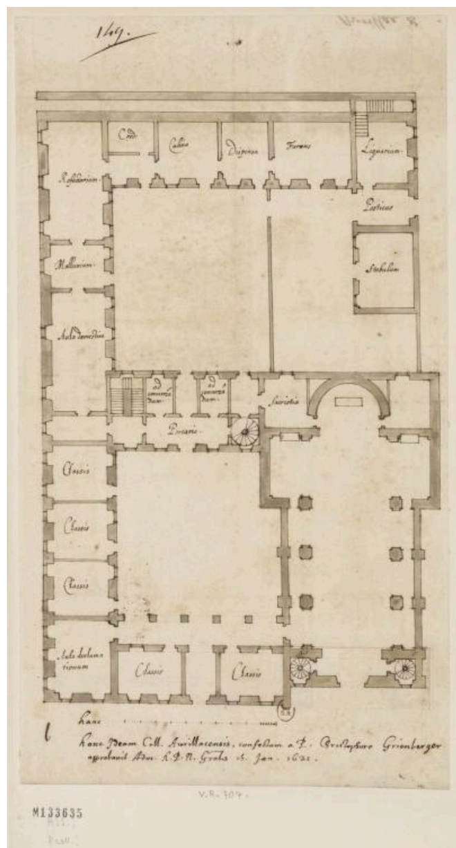
Plan du rez-de-chaussée, 2e projet, 1621 (B.n.F., Est., FOL-HD-4 (9))
