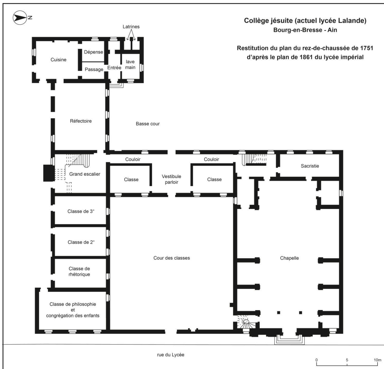
Rez-de-chaussée du collège des jésuites : schéma de restitution du plan d'après le devis de 1752 (Dess. Inv. G. Beuparland-Dupuis)
