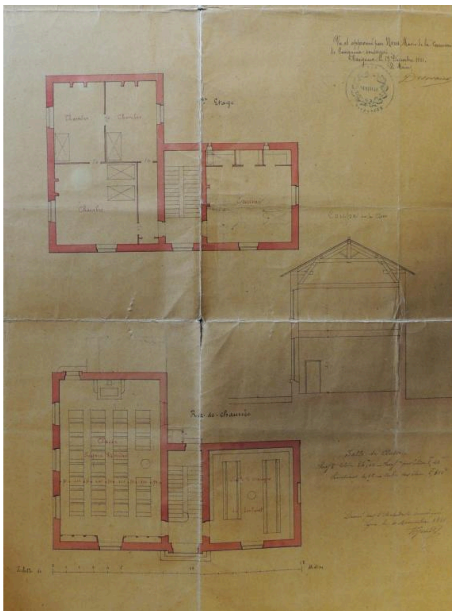
Maison d'école : plan, rez-de-chaussée, 1er étage, coupe, 1881 (AC Savigneux. M 1).
