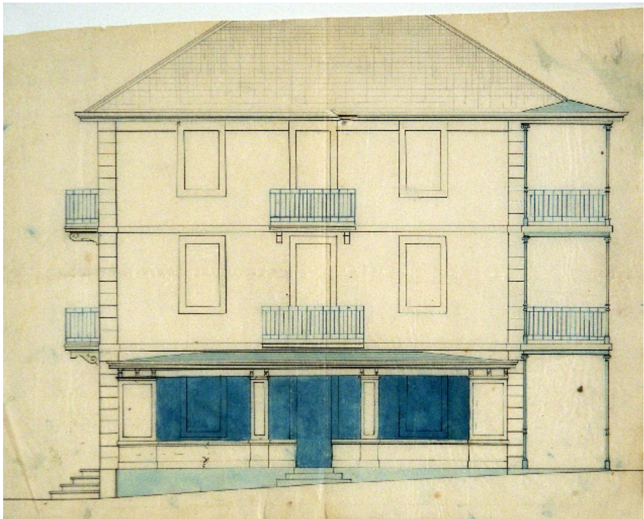
Elévation sud
