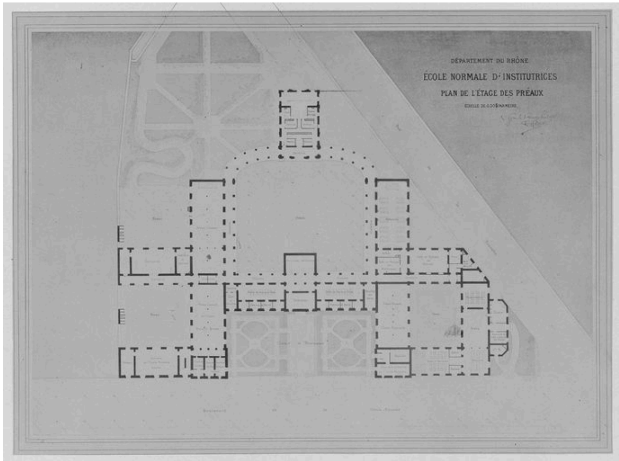
Plan de l'étage de soubassement de l'école normale (étage dit des préaux, 1888) (Arch. dép. Rhône, 1 T 1267, photographie de Fernique).
