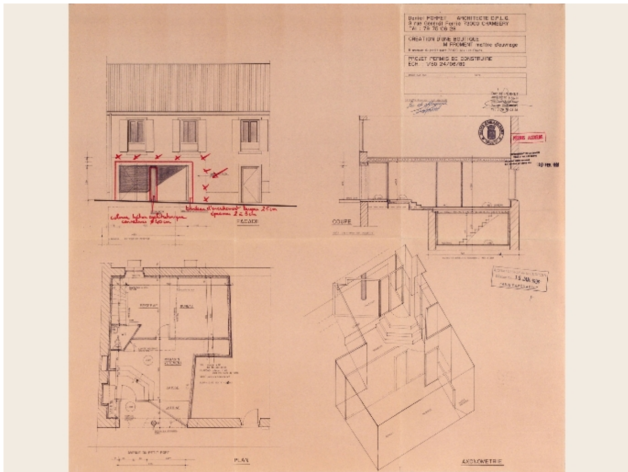
Plan, coupe et élévation du magasin
