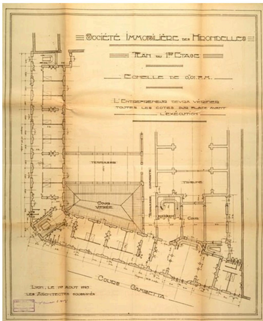
Plan du 1er étage / F. Chevallet et E. Martin, 1923 (AC Lyon. 344 WP 134)
