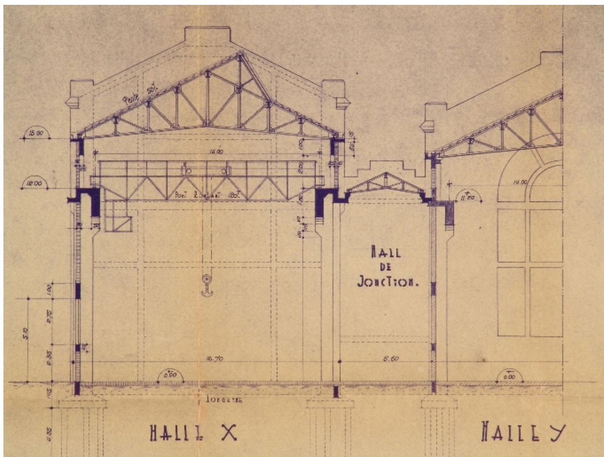
Coupe transversale de la halle X
