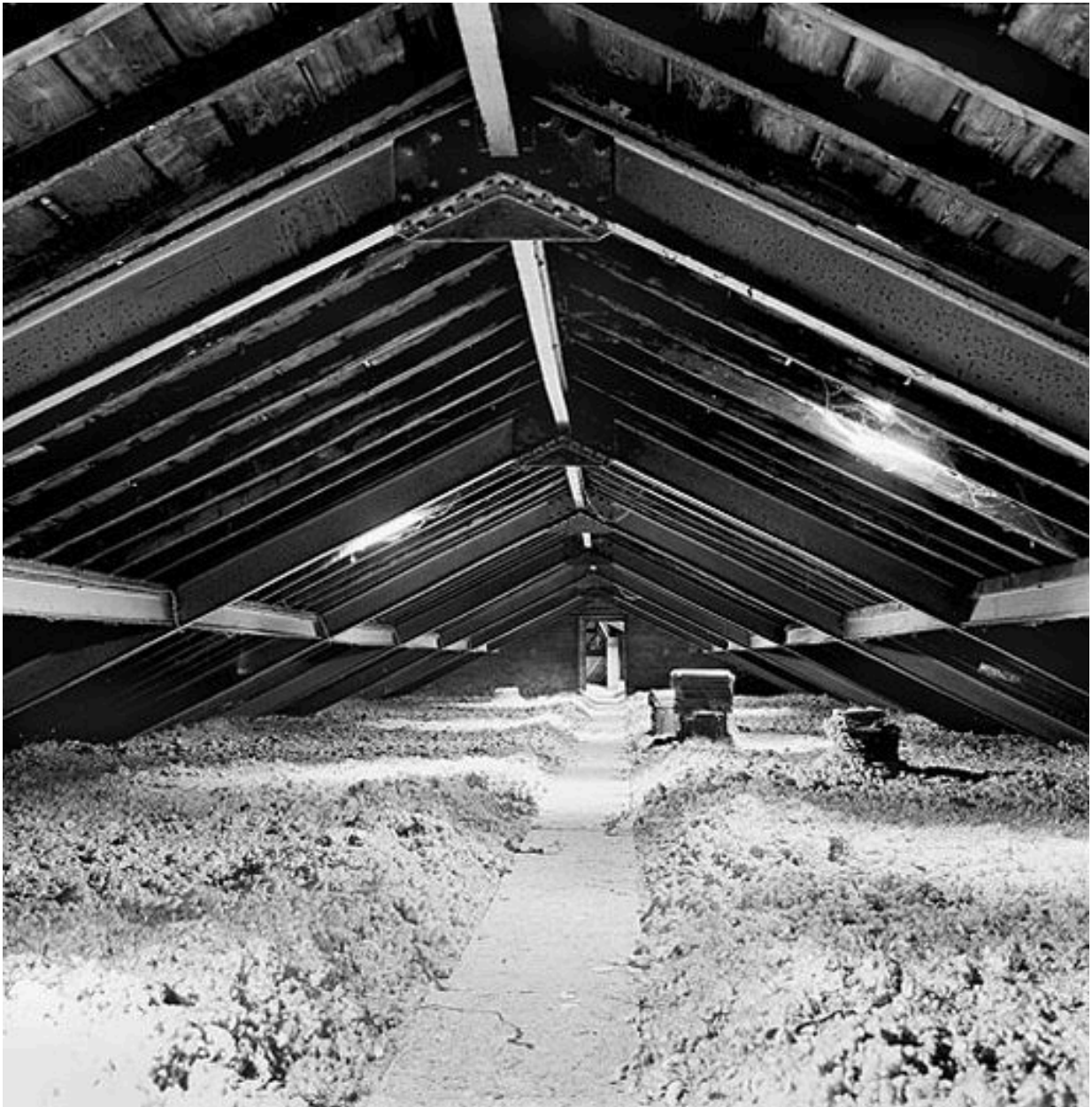
Charpente métallique des combles de l'ancienne école de filles, rue Gilbert-Dru
