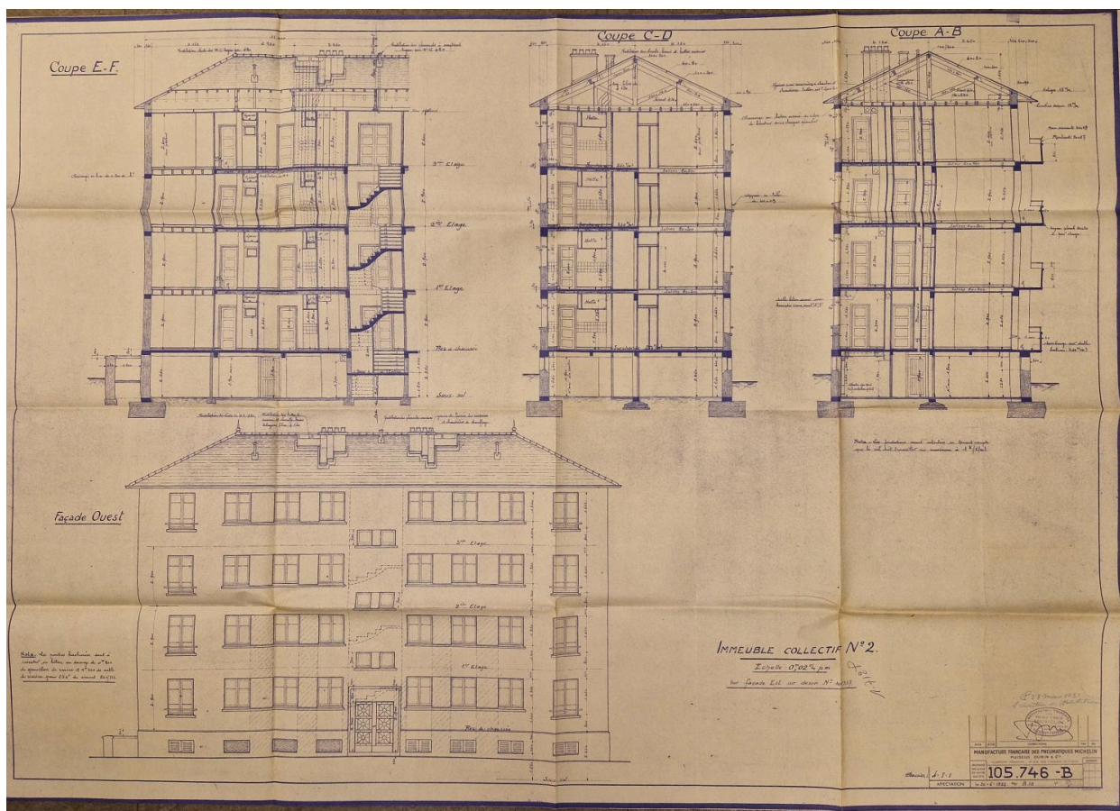
Projet d'immeuble au 42 bis rue de Blanzat : coupes et élévation ouest, 1952.
