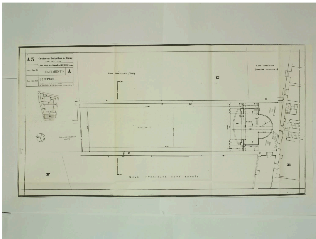
Plan, bâtiment A, 2e étage, éch. 002 p.m. État des lieux, septembre 1984.
