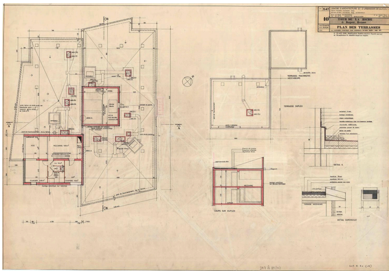
La Tour de la Biche, projet exécuté, plan des terrasses et du 22e étage (second niveau d'un appartement en duplex), février 1970, Faye et Tournaire architectes (AD63, 217 Fi 81 / 12).
