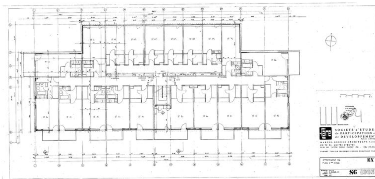
Plan du 2 e étage. Marcel Breuer, 3 février 1977 (AC Arâches-la-Frasse)
