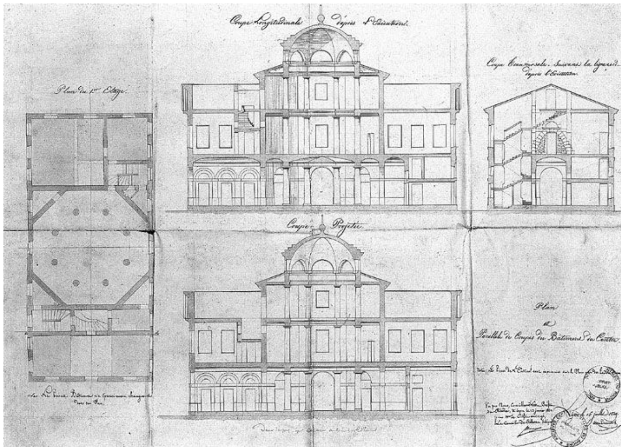
Plan et parallèle de coupes du bâtiment du centre, par l'architecte Dumont, 16 juillet 1829. 47,5 x 66 AD, Rhône. 1 Y 299
