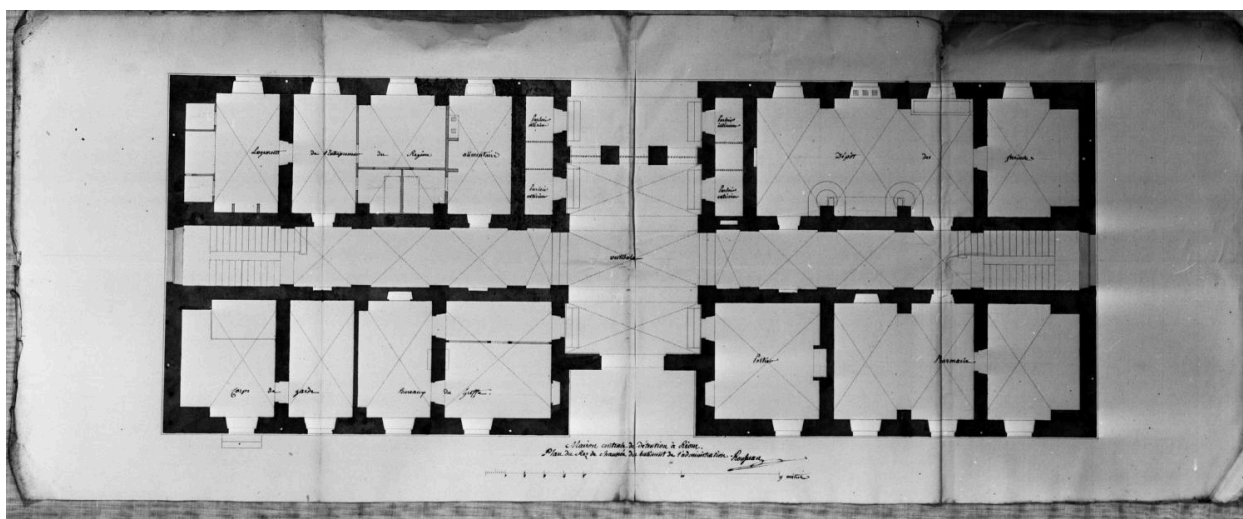
Maison centrale de détention à Riom. Plan du rez-de-chaussée du bâtiment de l'administration. Sans date, échelle en mètre, par Rousseau.
