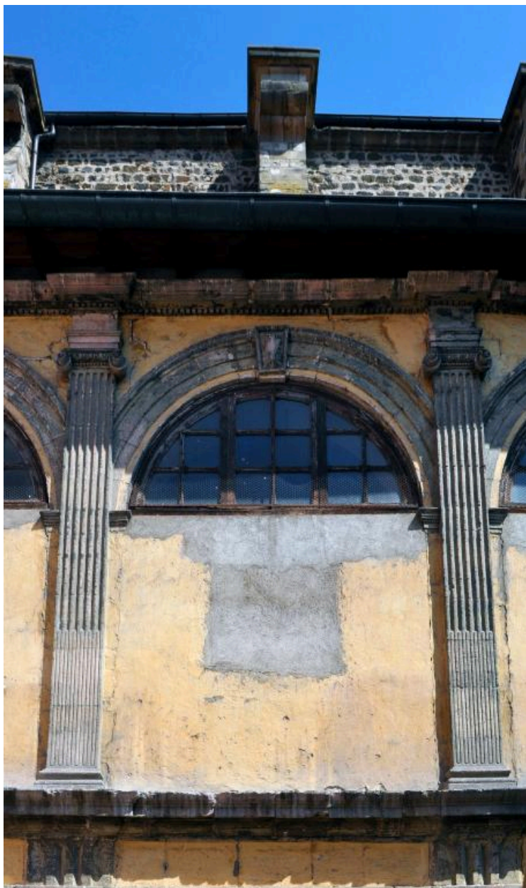
Galerie B : détail d'une travée
