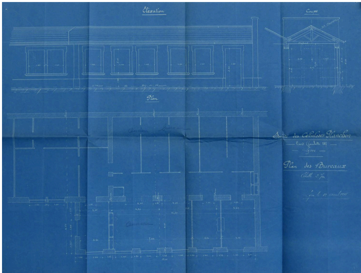
Plan des bureaux de l'ancienne usine Planchon cours A. Thomas (AC Lyon 314W/603)
