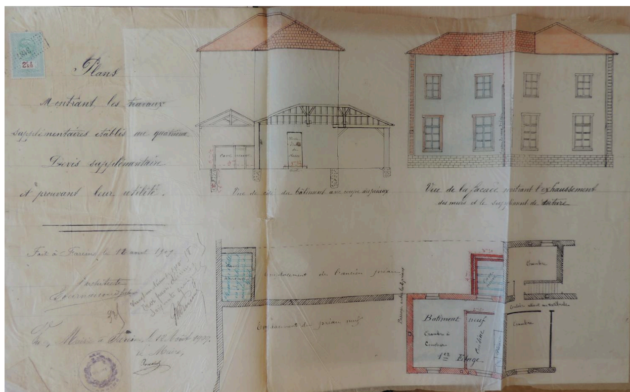
Plan pour l'agrandissement de l'école de filles, 1909 (AC Fareins, M 1).
