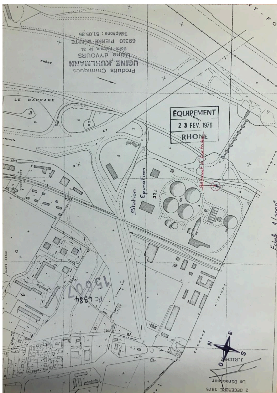
Plan de situation de la station d'épuration, 1976 (AC Pierre-Bénite : 203 – 68)
