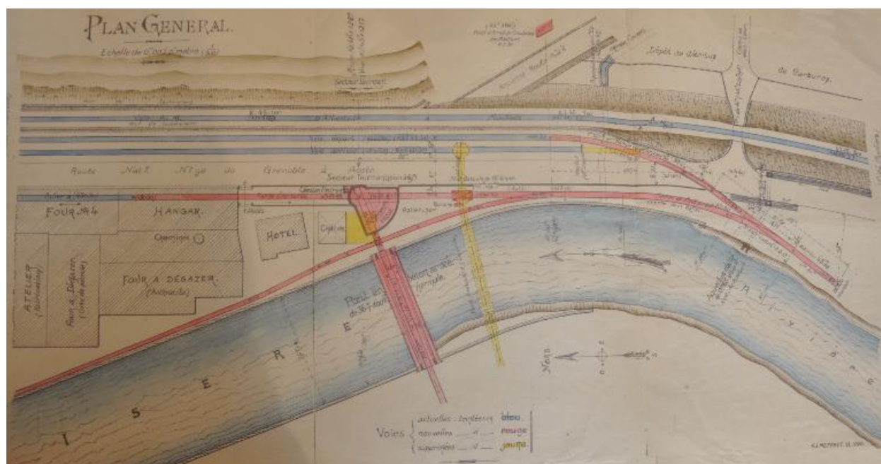
Plan des bâtiments de l'usine implantés en rive droite, 1920 (FR.AD073, 83S25).
