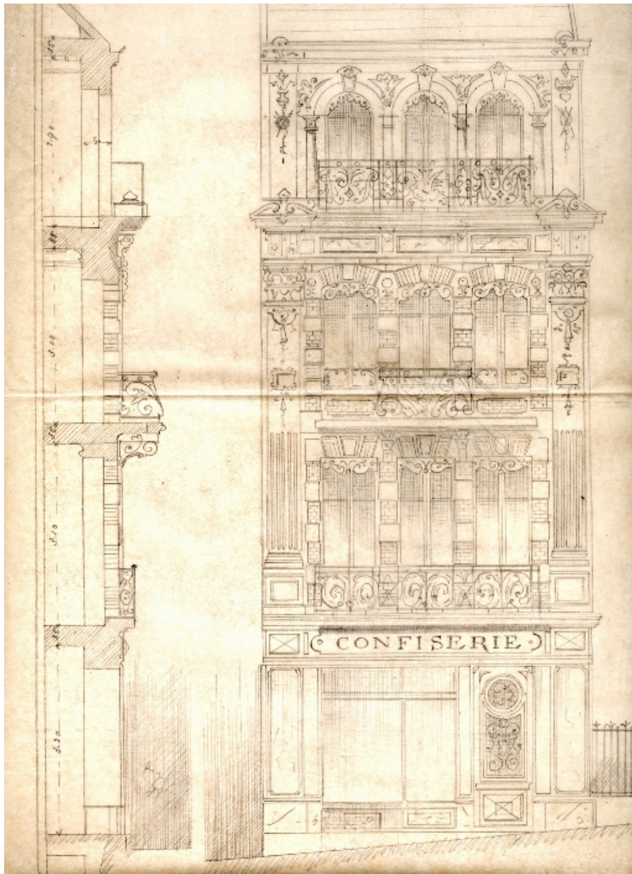
Elévation principale
