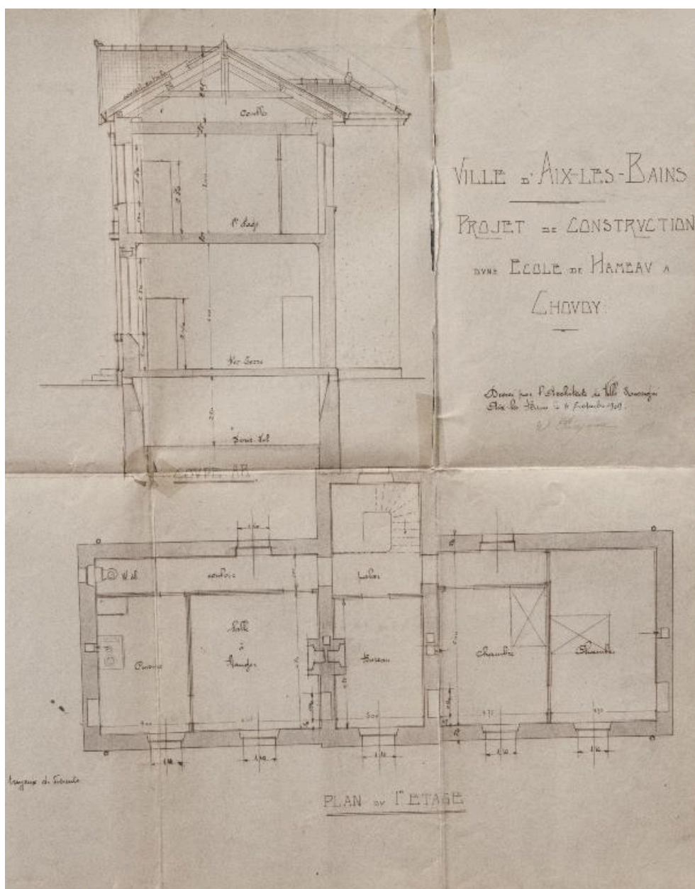
Plan de l'étage et coupe, 1909
