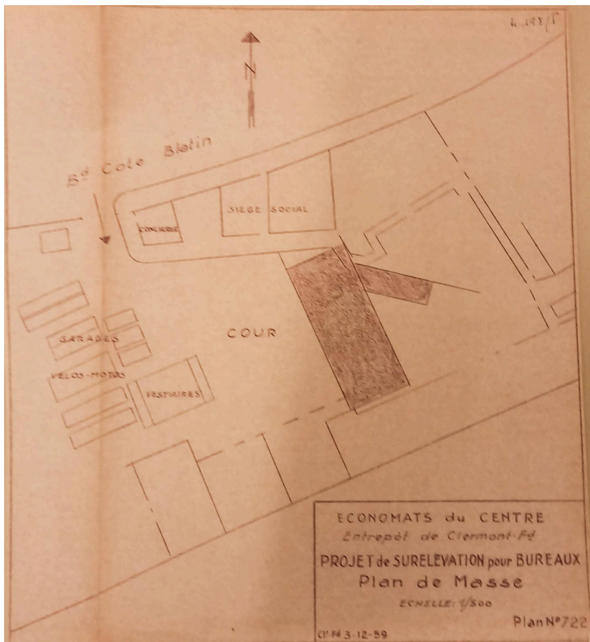
Plan de masse. Entrepôt dans la cour, 1959
