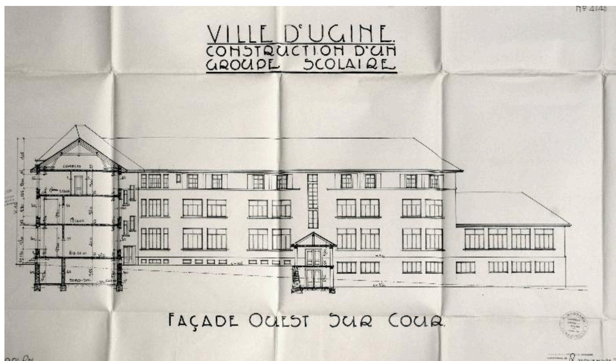
Ville d'Ugine, Construction d'un groupe scolaire. Façade ouest sur cour, Projet, A. Bugnard Novembre 1931 (AD Savoie, 2 O 2966)
