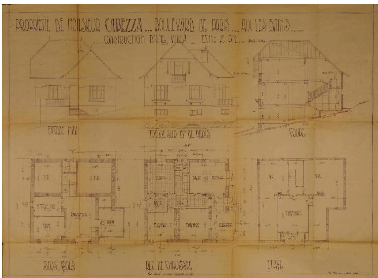
Villa Capezza, plans, façades et coupe, 1935
