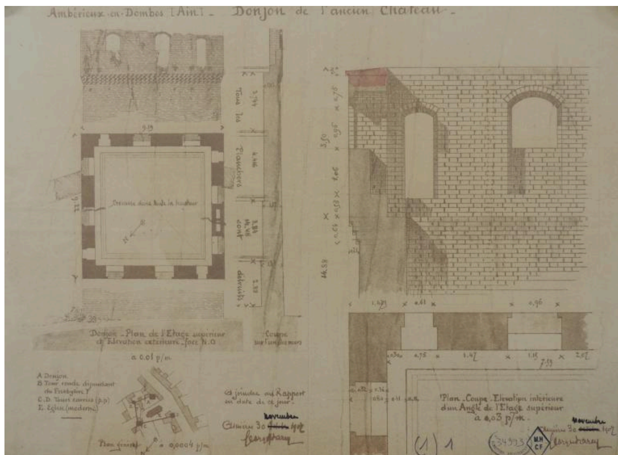
Plans, coupes et élévation intérieure du donjon. Georges Darcy. 1907 (MAP. 0082/001/2005).
