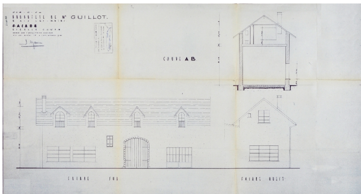
Elévations et coupe, 1955
