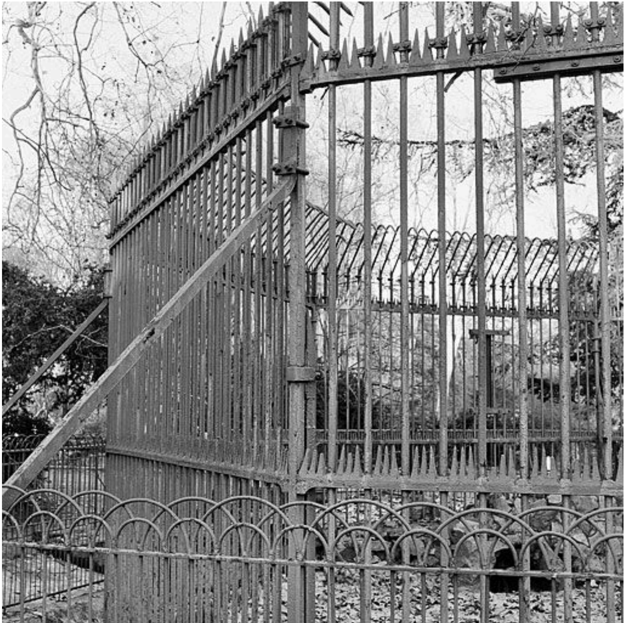
La cage aux ours : détail des assemblages
