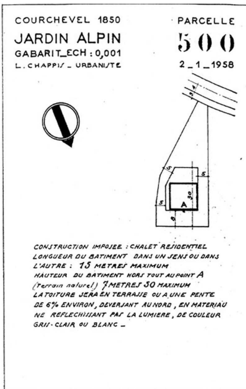
Chalet La Douna. Gabarit / L. Chappis, 2 janvier 1958.
