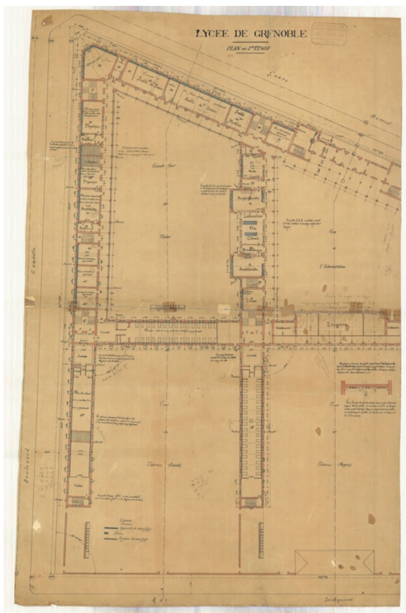
Plan du chauffage. 1er étage. 22 avril 1886.
