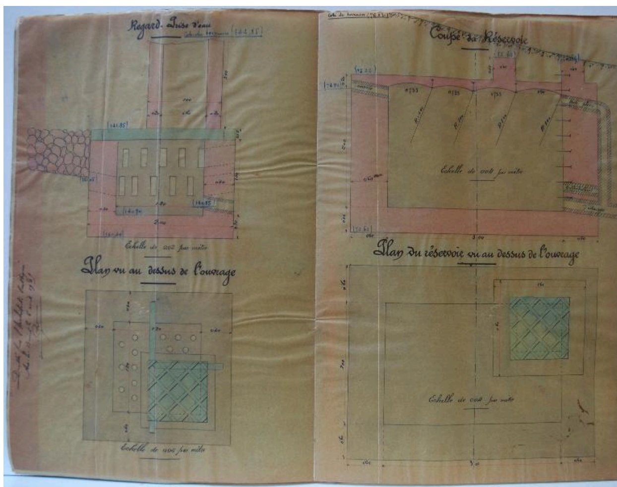
Ouvrages d'art projet d'aménagement d'eau, 1905. Réservoir, regard.
