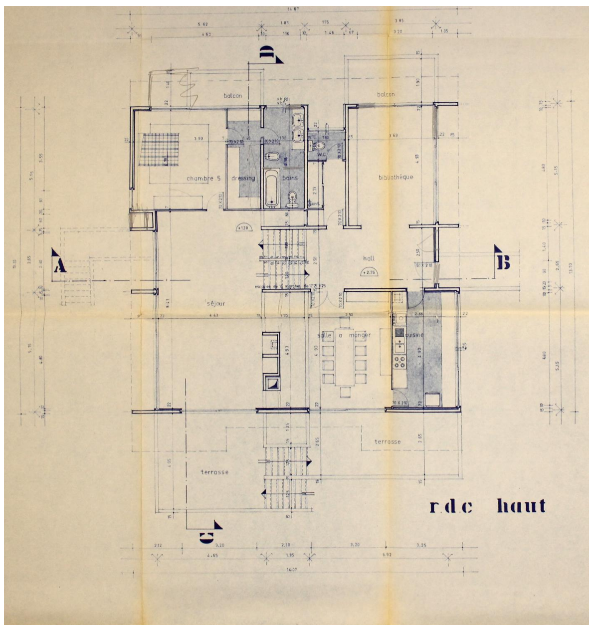
Clermont-Ferrand, la villa F., plan du rez-de-chaussée haut, Michel Vigneron architecte, 1969 (archives municipales de Clermont-Ferrand).
