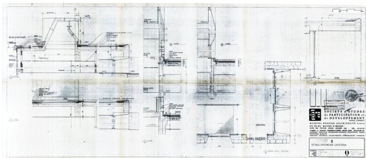
Appartement Q. Cafeteria. Détails des murs extérieurs. Marcel Breuer architecte, 30 novembre 1969 (AC Arâches-la-Frasse)
