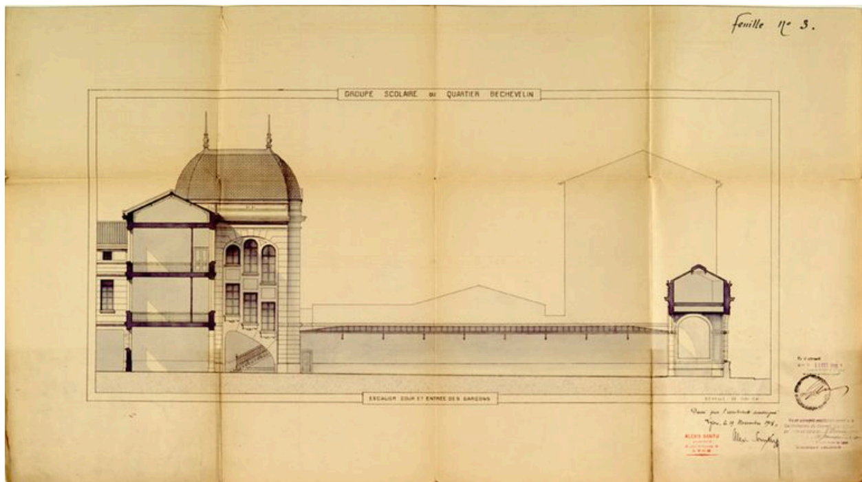
Escalier, cour et entrée des garçons. Elévation, 1908. Dessin à la plume (AC Lyon. 0476 WP 53)
