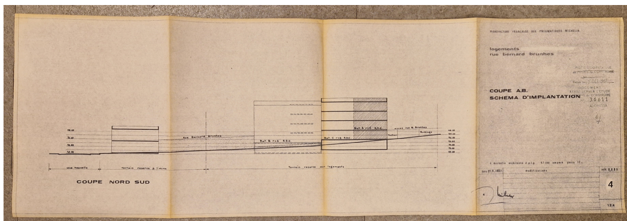
Coupe nord-sud des bâtiments de la rue Bernard Brunhes, par Daniel Michelin, 1967.
