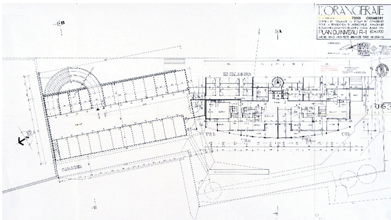
Plan du 2e étage de soubassement
