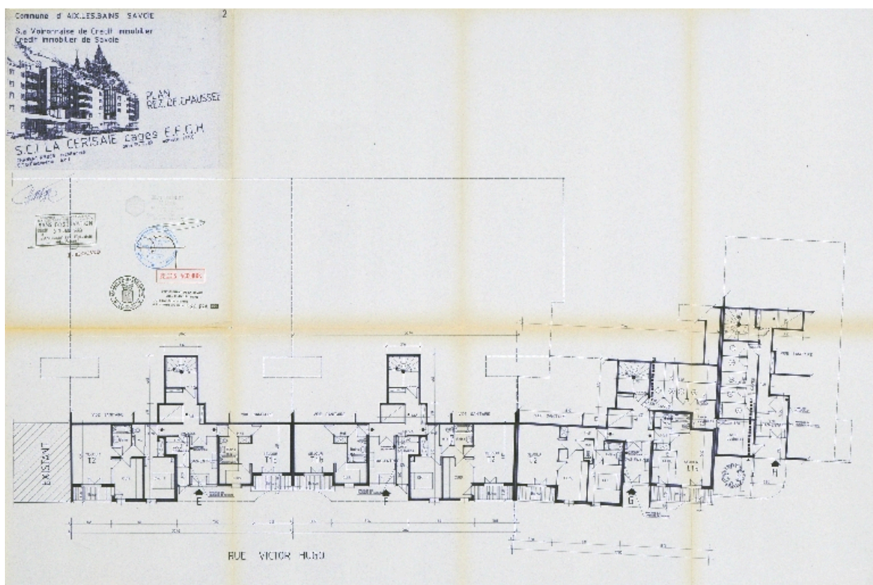
Plan du rez-de-chaussé des cages E, F, G et H
