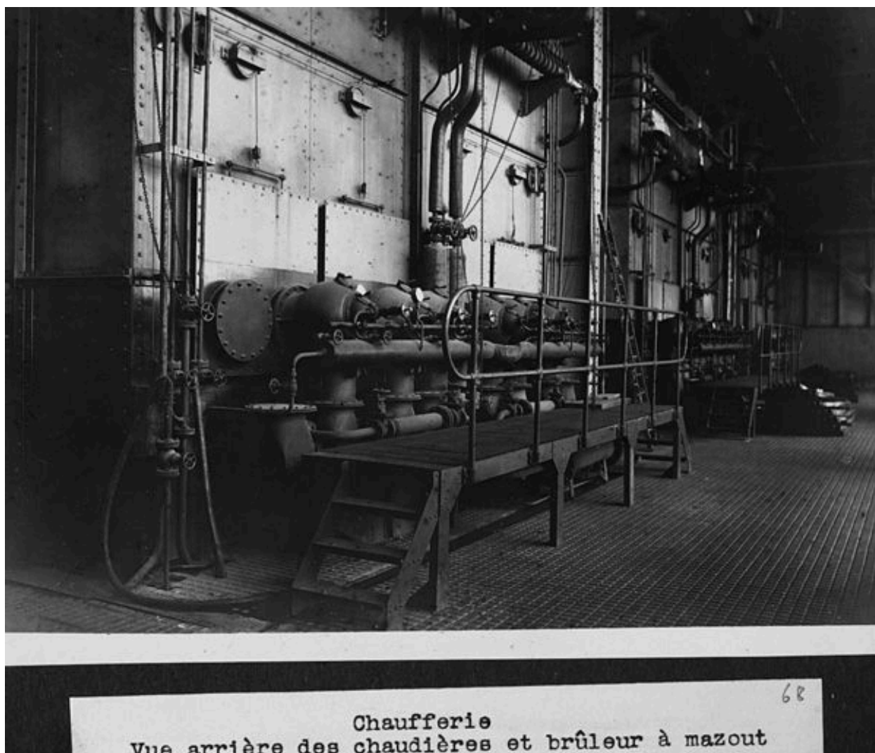
Chaufferie. Vue arrière des chaudières et brûleurs à mazout. Photogr., vers 1960
