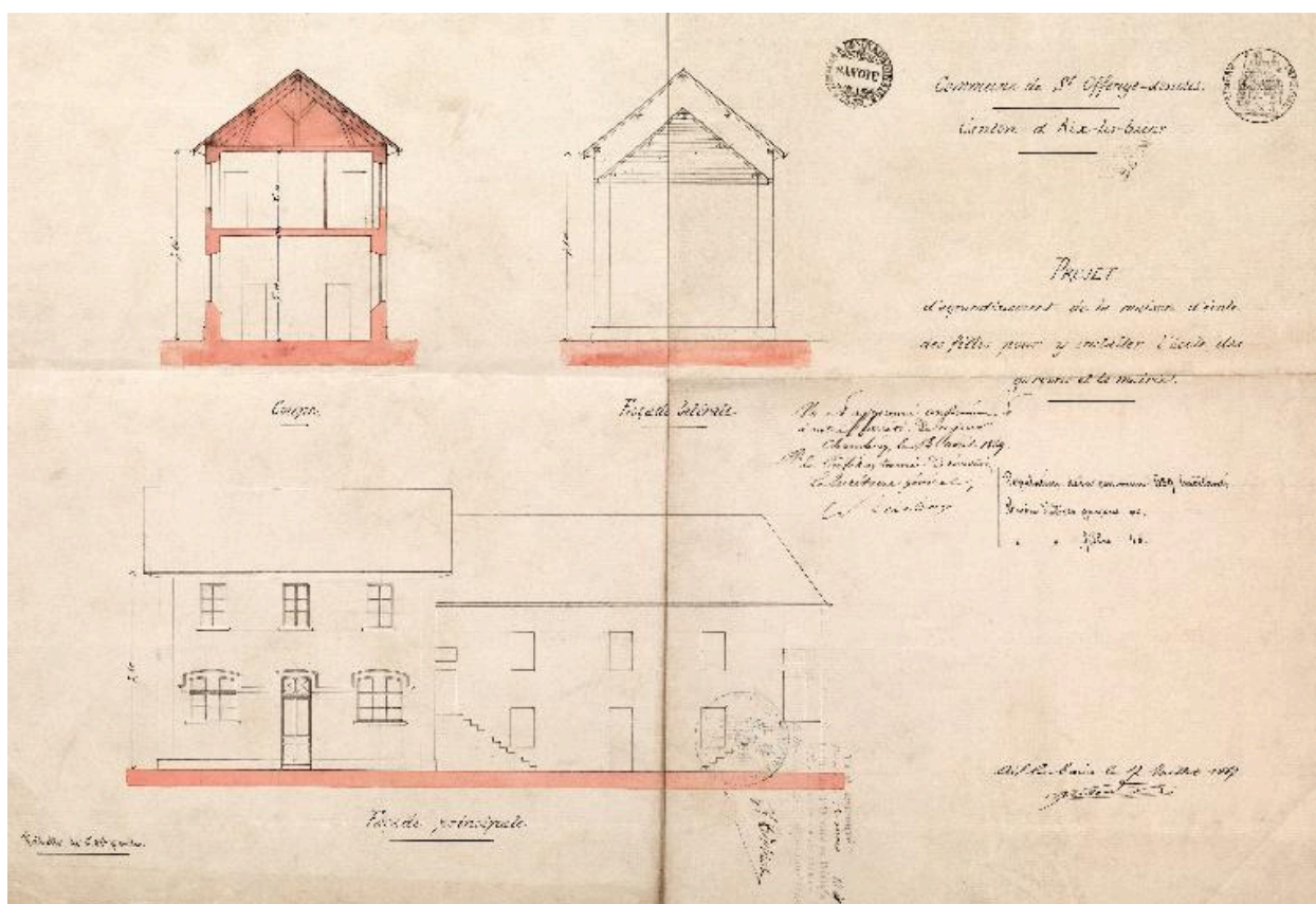
Projet d'agrandissement de la maison d'école des filles pour y installer l'école des Garçons et la mairie. Coupe, Façade latérale, Façade principale. Grisard, 1867.
