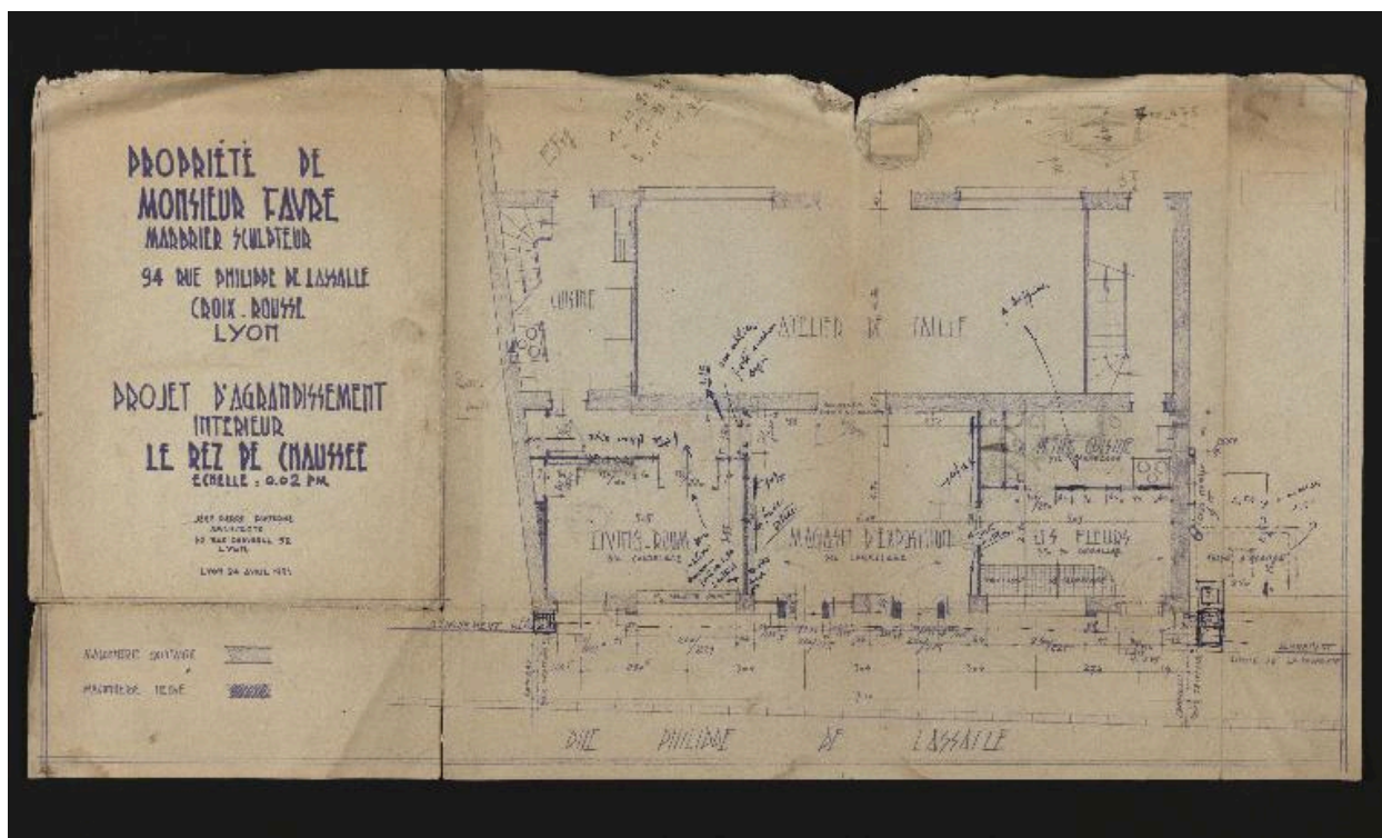
Plan du rez-de-chaussée : projet d'agrandissement intérieur, Jean-Pierre Fonterme architecte, 24 avril 1951
