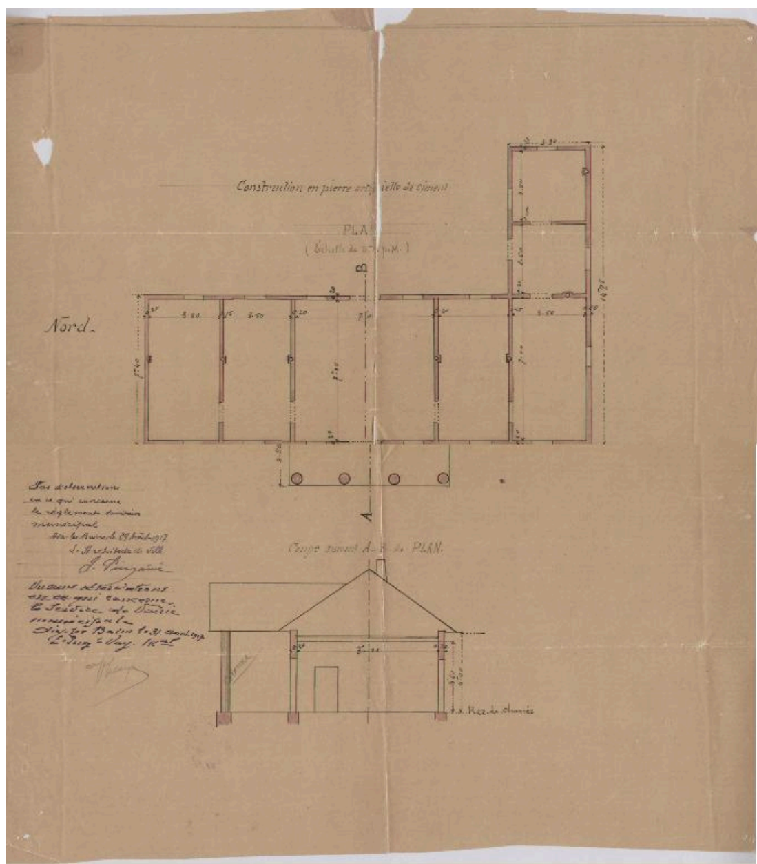
Plan et coupe, 1917
