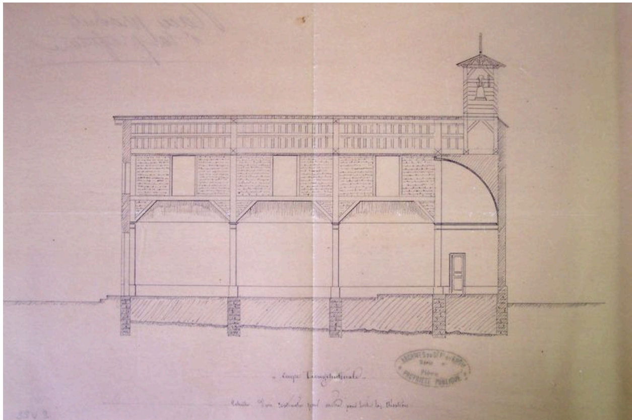
Coupe longitudinale par Bourdet
