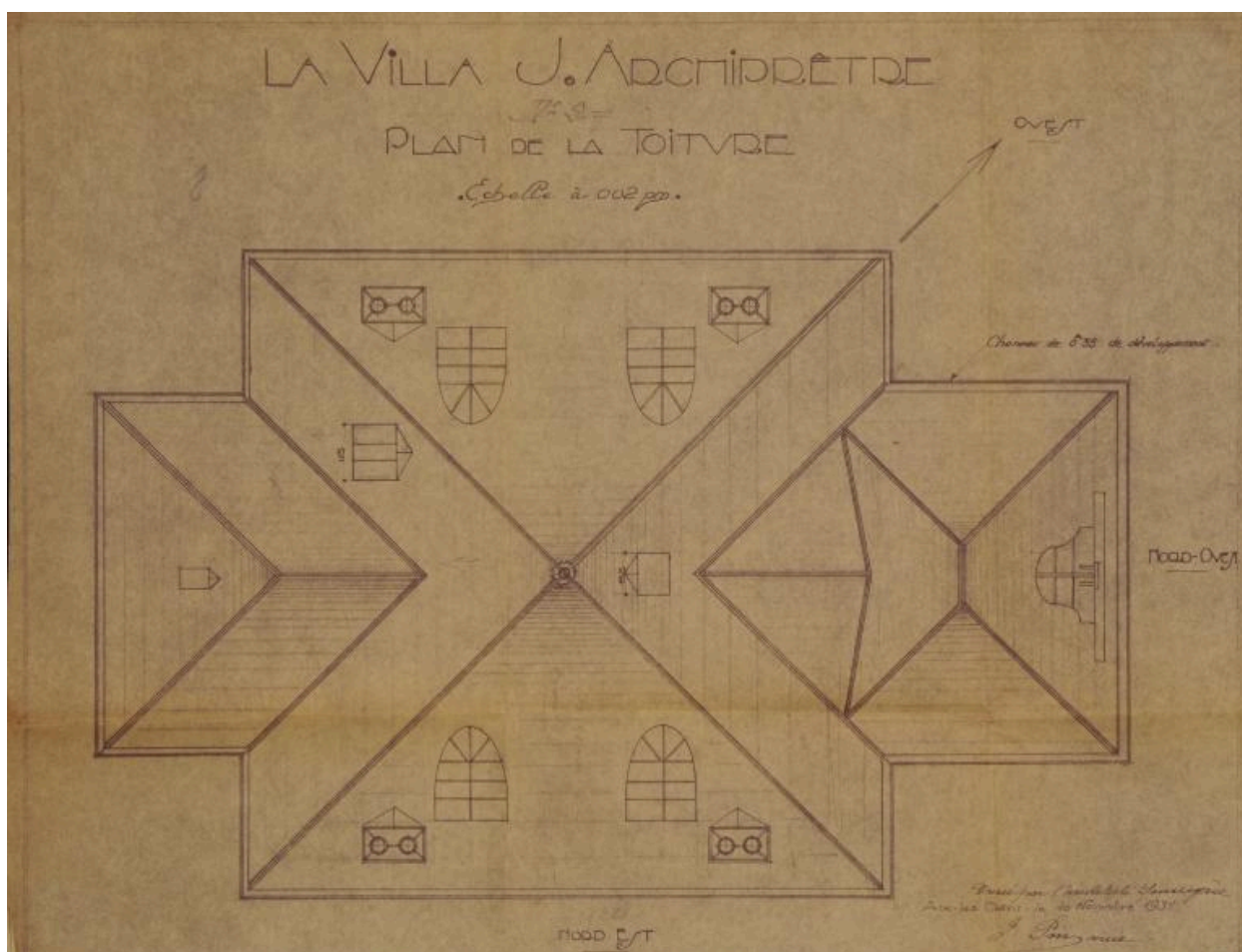
Plan de la toiture, 1931, projet non réalisé
