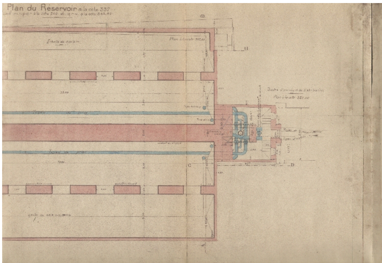
Plan du réservoir, partie droite
